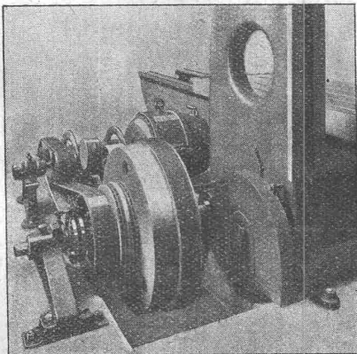
Hobelmashinen-Einzelantrieb mit elektro- magnetischer Reversier-Reibungskupplung Patent Clus und Umkehr-Lnix.
