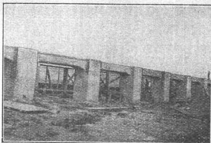
Fundationsarbeiten des Grenzbahnhofes Lüttenburg (Dep. Bas-Rhin)
