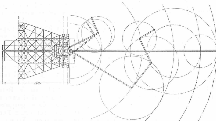
Abb. 19. Schema der Gussbeton-Anlage auf der Schleusen-Baustelle. (Nach „VDI-Zeitschrift“.)
