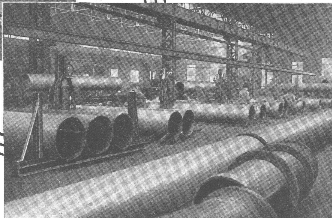
1600 Meter autogen geschweißte Rohre aus Armco Eisen, 600 mm Durchmesser, für das Ministerium für Öffentliche Arbeiten, Kairo.
