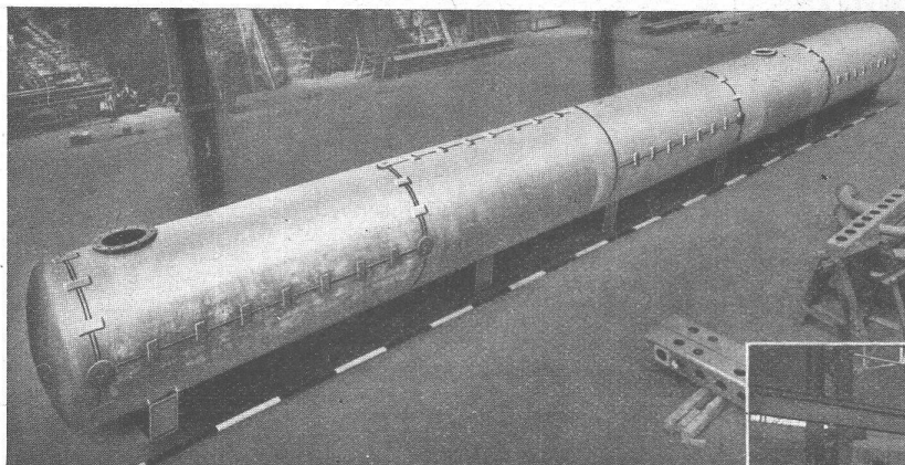
Mehrere dieser Kondensat-Kessel stellte die Firma L. u. C. Steinmüller, Gummersbach, aus Armco Eisen her. Die Verbindungen wurden mit Armco Eisen-Draht elektrisch geschweißt.
