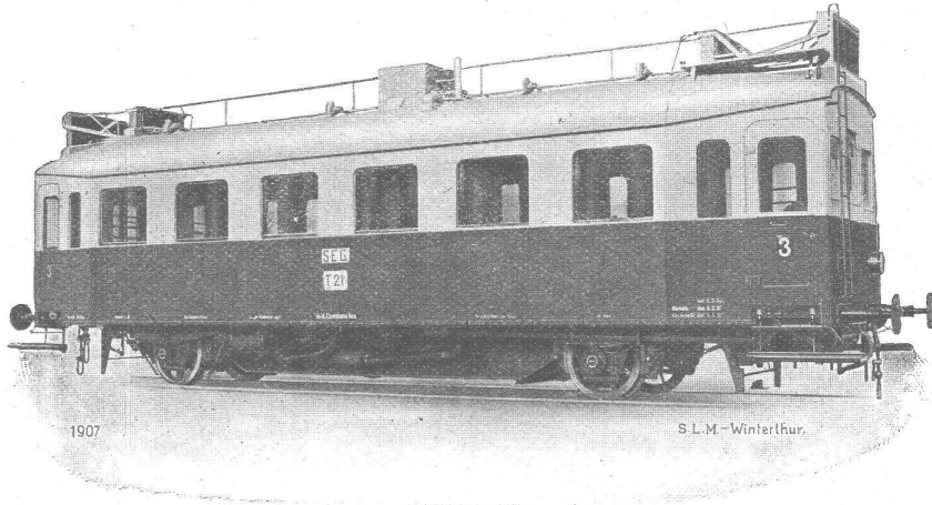
Dieseltriebwagen von 130 PS Leistung der Süddeutschen Eisenbahn-Gesellschaft Darmstadt, ausgerüstet mit einem kompletten vierstufigen Antrieb System „S. L. M.-Winterthur“.
