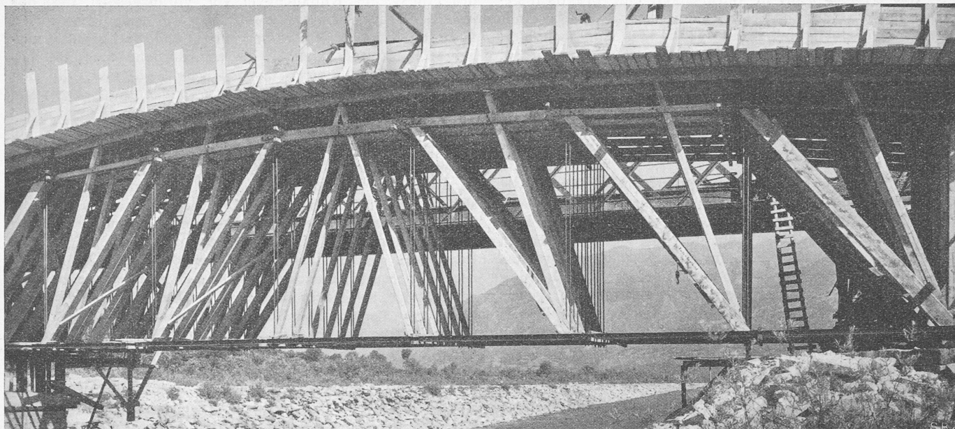
Abb. 4. Einzelheiten des Lehrgerüsts (1930) nach System Klinker & Meyer, Ingenieurbureau, Zürich.
