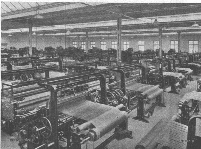
Brown Boveri-Rüti Zahnradantrieb für Seidenstühle.
