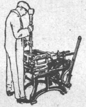
Handbedienung 300 Blöcke und Hohlblöcke od. 1500 Steine täglich
