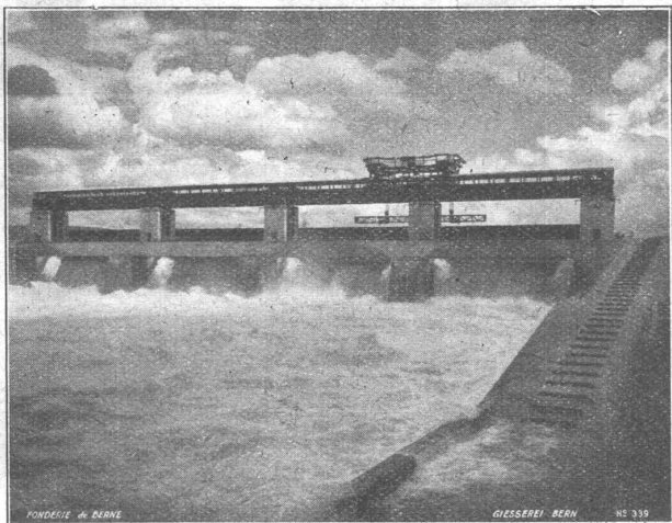
Stauwehr Ryburg-Schwörstadt.
