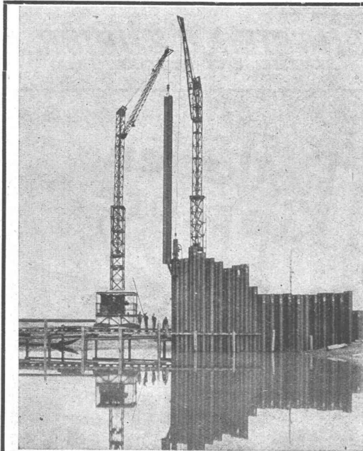
Rahmen von „Larssenwänden“ Kraftwerk Klingnau
