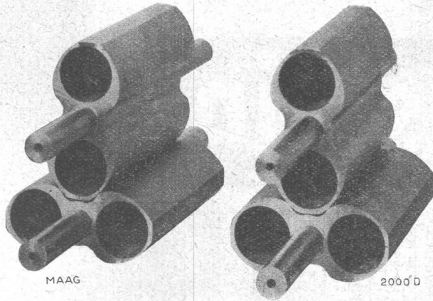
KOMPRESSORENFLÜGEL mit nach besonderem Verfahren genau bearbeiteten Evolventenzähnen.
