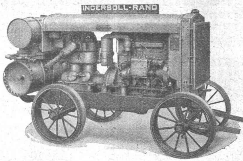
Rohölkompresseur 20/26 PS.
