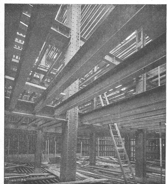
Tresorkonstruktion eines Bankgebäudes
