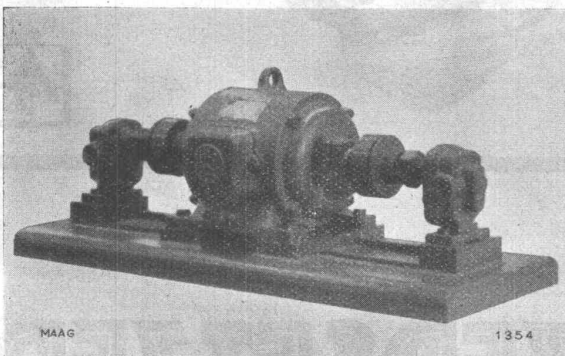
MAAG-ZWILLINGSZAHNRADPUMPE zur Erzeugung eines Oeldruckes von 50 at in einer Doppelpresse. Beide Pumpen geben auf 1 % genau gleiche Drücke und Förder- mengen.
