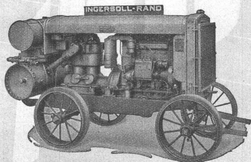
Rohölkompressor 20/26 PS.
