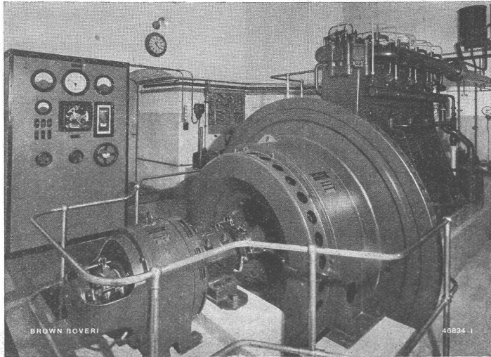
Automatische Notstromgruppe 250 kVA in einer Radiosendestation
