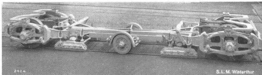
Drelachsiges Motorwagen-Untergestell der Strassenbahn Zürich
