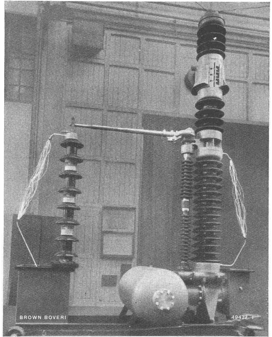
150 - kV - Druckluftschneiderschalter Prüfung mit Stossspannung
