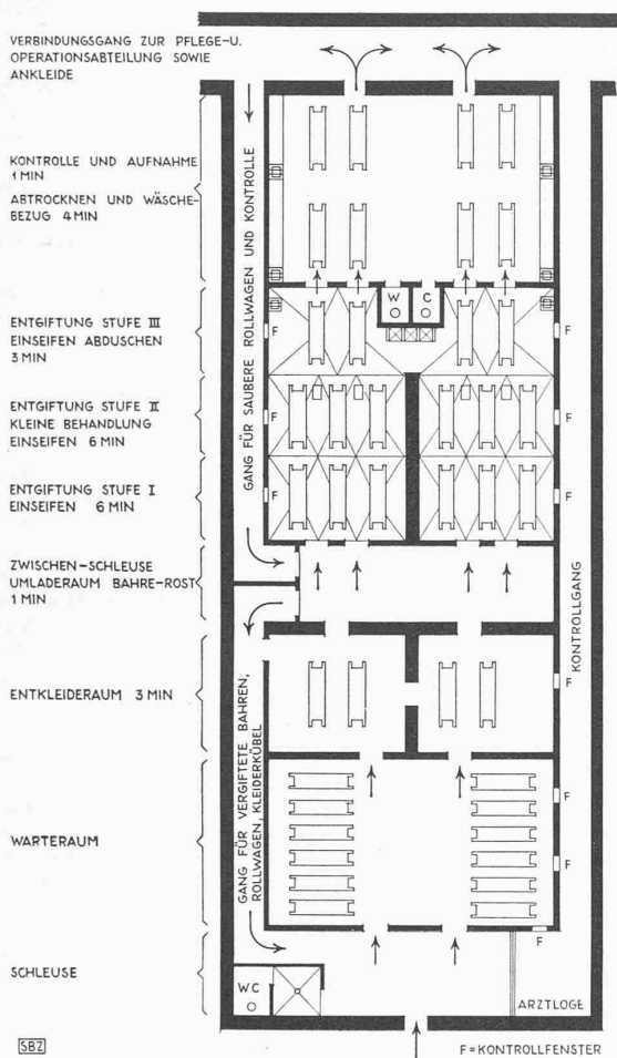
Schema (1:300) einer Entgiftungsanlage für 2x30 bahrenlägrige Patienten pro Stunde. Dipl. Arch. F. LODEWIG, Basel
