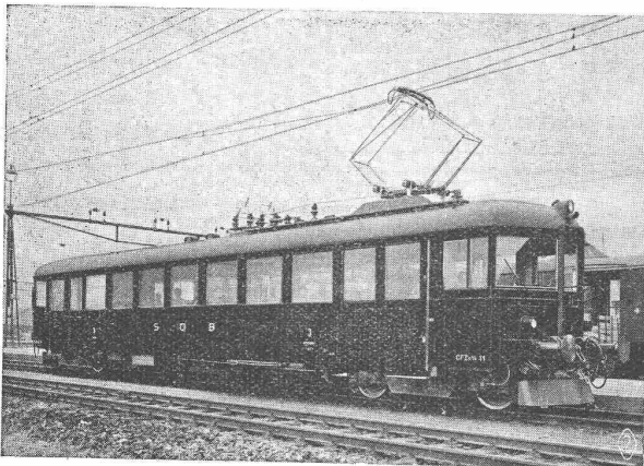
Sämtliche 8 Triebwagen der neu elektrifizierten Südostbahn wurden mit elektropneumatischen Sécheron-Hüpfsteuerungen ausgerüstet
