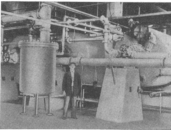
Extraktionsanlage für Gewinnung von Salatöl aus 50 t Maiskeimen täglich, in den USA.
