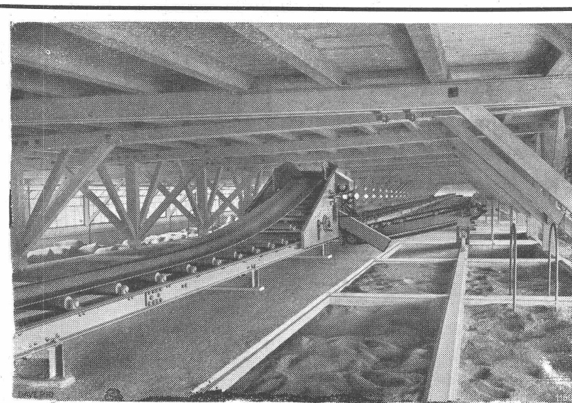
Transportanlage für loses und gesacktes Getreide in einem schweizerischen Lagerhaus
