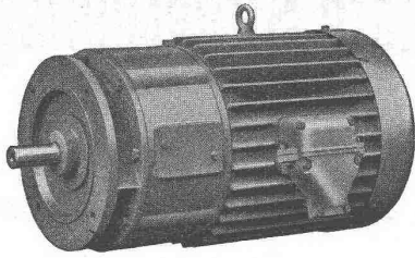
Als Flanschmotor, geschlossen mit Oberflächen-Rippenkühlung.
