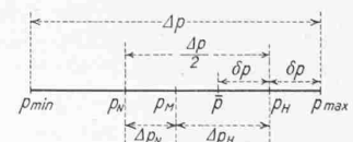
Abb. 5. Druckverhältnisse bei Schaltung I
