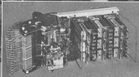
EINSTELLUNG DER HEBDREH- WÄHLER-KONTAKTFEDERN
