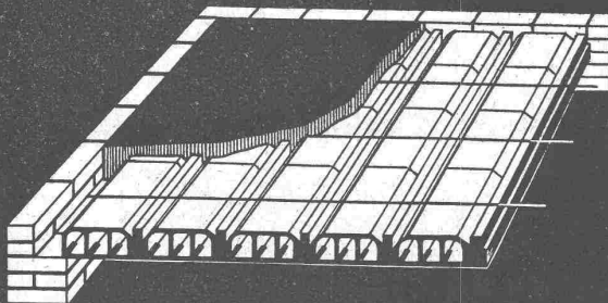
Schalungslose Steghohlkörper-Decke
