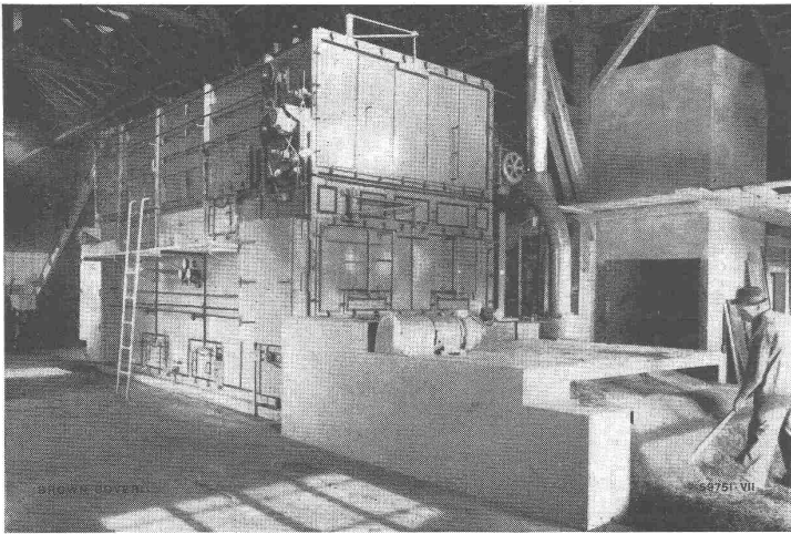
Grossgrastrockner-Anlage, Grastrocknungs-Genossenschaft Burgistein, Kt. Bern
