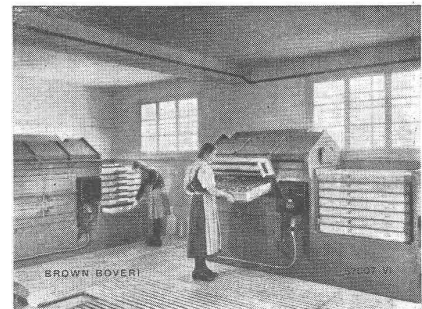
Zwei elektrische Universal-Trockner, Landwirtschaftliche Konsumgenossenschaft Gontenschwil, Kt. Aargau
