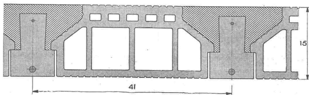
Decken-Querschnitt bei Verwendung der zementsparenden Spezial-Deckensteine
