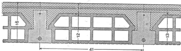
Decken-Querschnitt bei Normal-Ausführung
