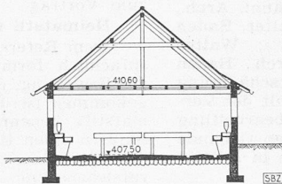
QUERSCHNITT DURCH BRUTRAUM
