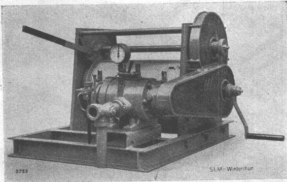
Seilwinde mit Rotations-Druckluftmotor
