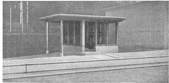
50t Geleisewaage mit armerter Betonbrücke, torsionsfreien Hebeln und verstellbaren Schneiden
