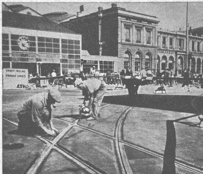
Umbau Bahnhofplatz, Einbauen von Fugenkitt PALTOX zwischen Tramgeleise und Strassenbelag
