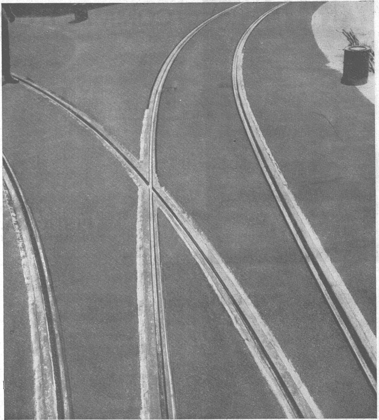
Umbau Bahnhofplatz Zürich, Einbauen von Fugenkitt-Paltox zwischen Tramgeleise und Strassenbelag
