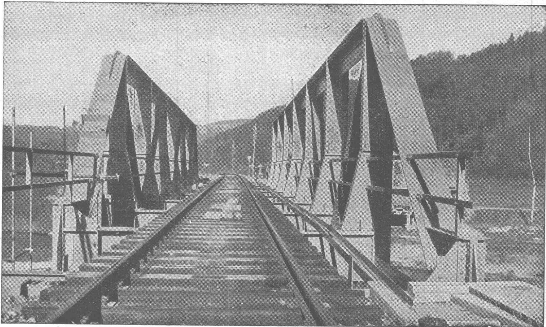
Tössbrücke Wila
