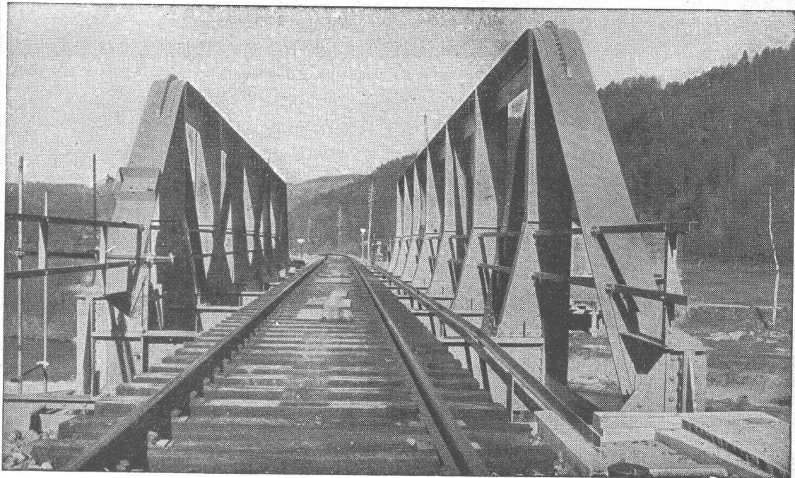
Tössbrücke Wila
