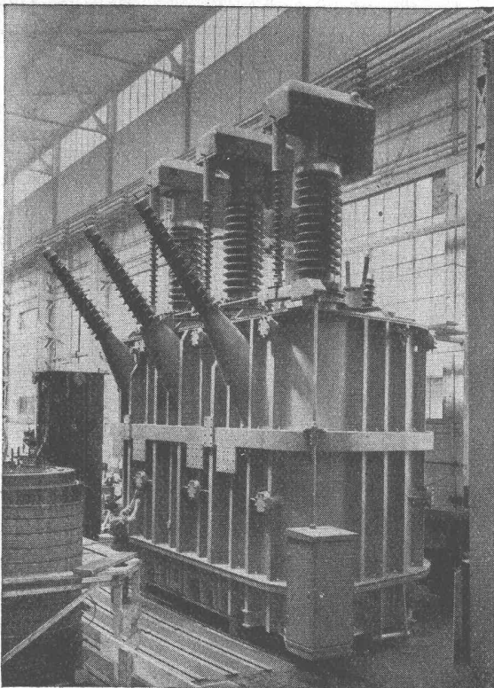
Drehstrom-Transformator von 50 000 kVA Bestimmungsland: Algerien
