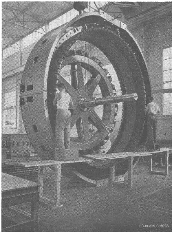
Kraftwerk Vittingfloss - Norwegen Stator eines Drehstromgenerators von 5400 kVA, 5000 V
