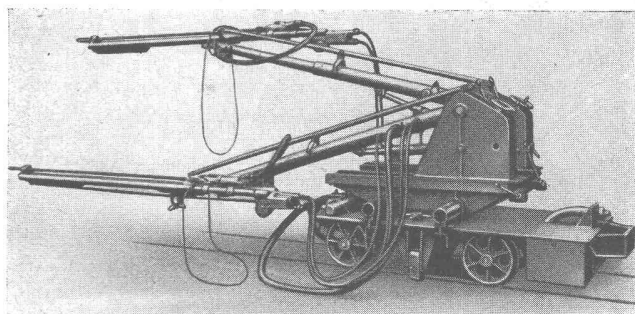
BOHRWAGEN für schlagendes und drehendes Bohren zur Erleichterung und Verkürzung der Bohrarbeit
