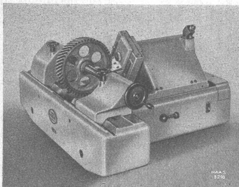
Zahnschrägemessgerät, Typ HM-30, für Stirn- und Schraubenträger bis 300 mm Durchmesser.
