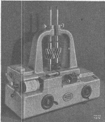
Achsdistanz- und Rundlaufprüfgerät, Typ DAS-10, für Stirn- und Schraubenträgerpaare bis 120 mm Achsdistanz.
