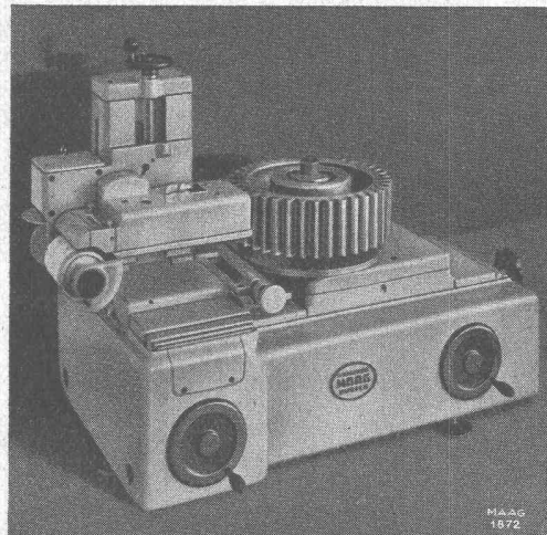
Zahnschrägemessgerät, Typ HM-30, für Stirn- und Schraubenträger bis 300 mm Durchmesser.
