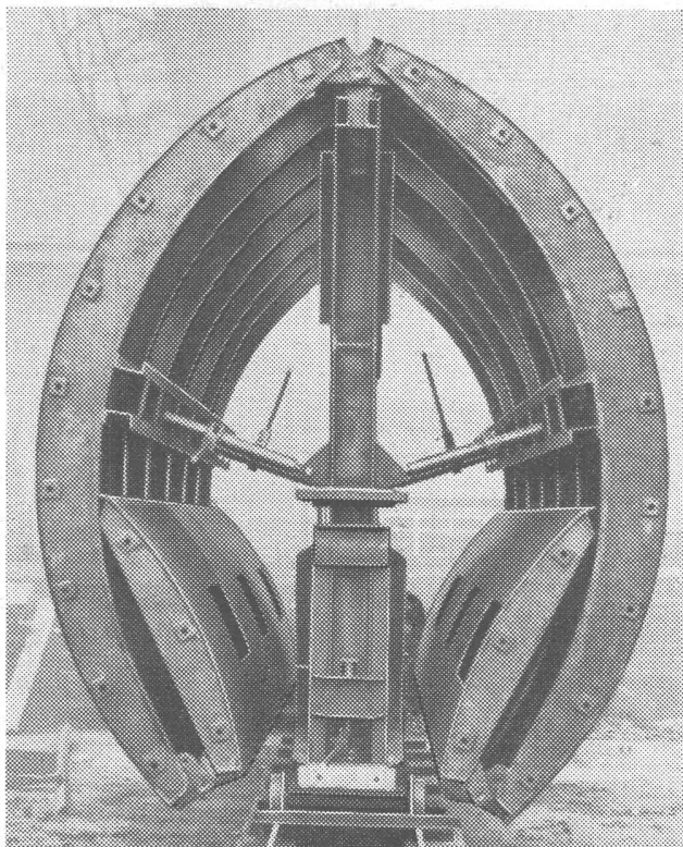
Teleskop-Stollenschalung \phi 3,75 m auf Transportwagen
