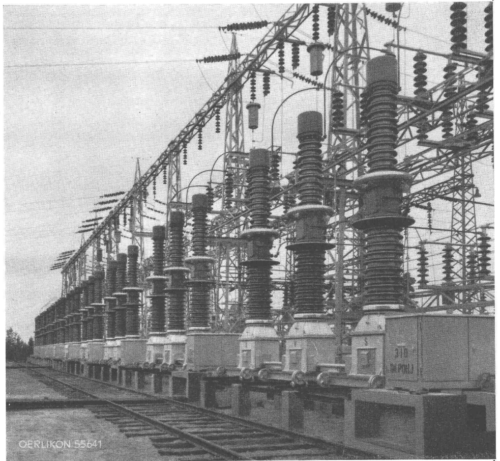
Gruppe von 9 ölarmen Schaltern, Typ TOF, 135 kV, 2500 MVA, in einer Transformatorstation in Finnland.
