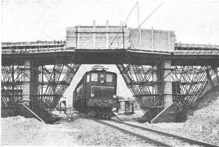
Lehrgerüst Strassenüberführung bei Schwerzibach für Fa. W. Küenzi, Lachen
