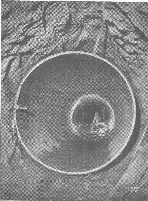
Druckschacht-Panzerrohr in Montage. Durchmesser 2,2 m. Betriebsdruck 33 at.
