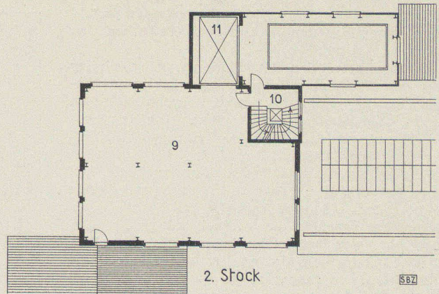
Bild 8. Zweiter Stock 1:400
