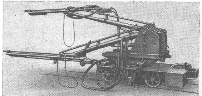
BOHRWAGEN für schlagendes und drehendes Bohren zur Erleichterung und Verkürzung der Bohrarbeit
