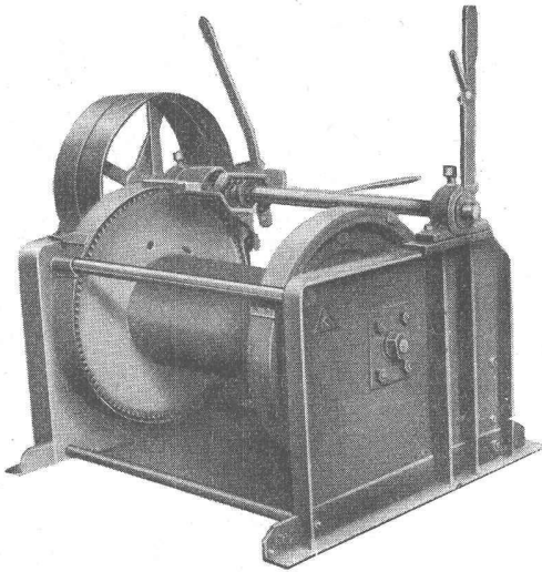
Seilwinde KS 23/70 mit gefrästem Stirnradgetriebe
