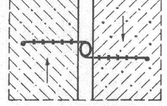
Bild 4. Scherbeanspruchung (Setzung)
