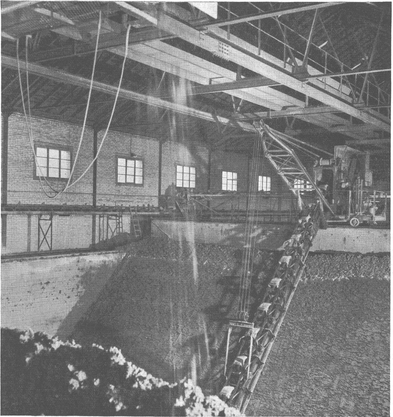
Lehmaufbereitung und automatische Mischung in der Sumpfanlage
