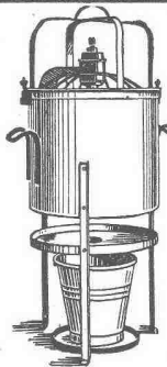
Exsiccator für Neubau- Austrocknung
