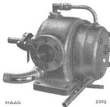
Hochdruck-Innen- verzahnungspumpe für hydraulische Steuerungen. Druck bis 200 atü
