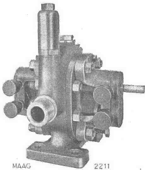
Zahnradpumpe für Seifenwasser, Fruchtsäfte, Benzin etc.
