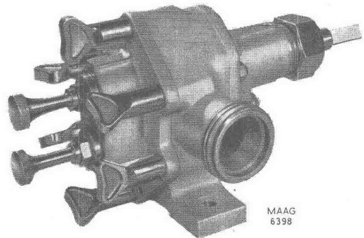
Zahnradpumpe zur Förderung von Milch, Rahm und Kondensmilch
