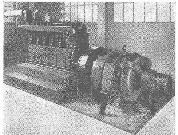
Diesel-Generator-Gruppe 600 PS, störungsfrei isoliert
