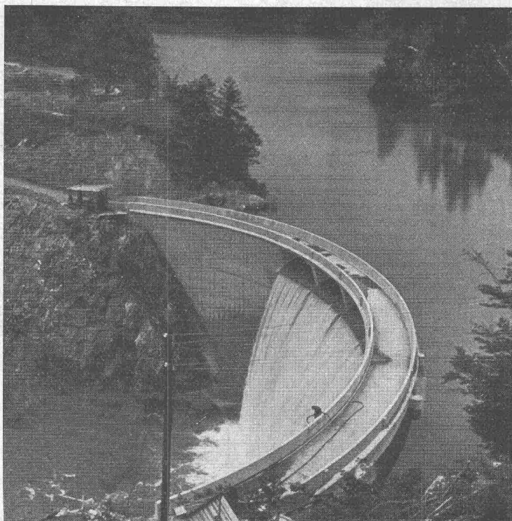
Weissenseesperre, Kraftwerk Kamering (Kärnten), erbaut durch die KELAG in FRIOPLAST-Beton
