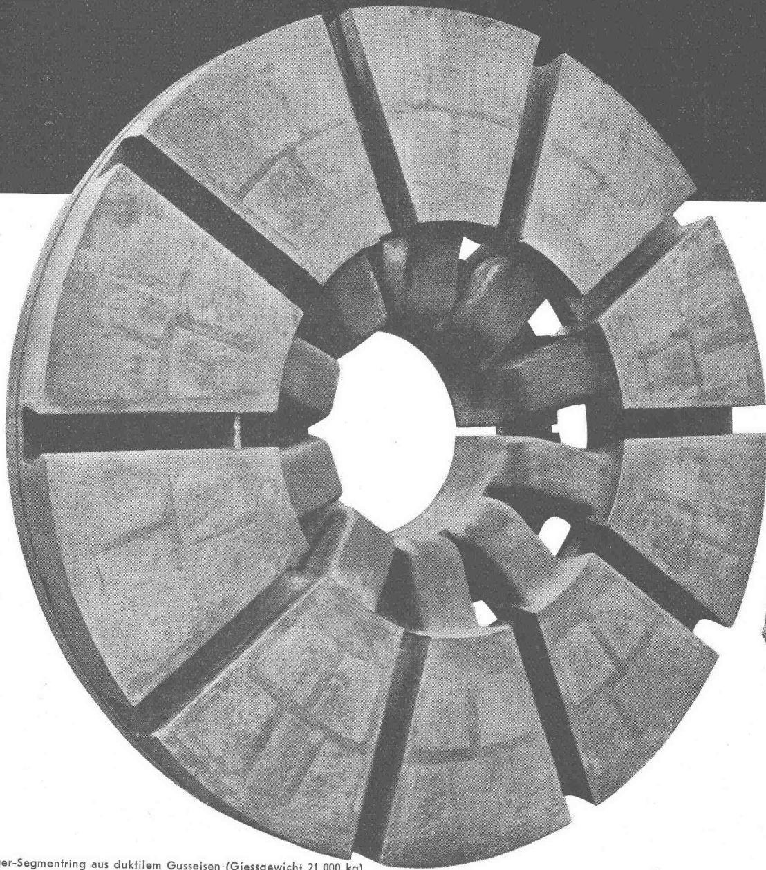
Spurlager-Segmentring aus duktilem Gusseisen (Giessgewicht 21 000 kg) für eine Kaplanmaschine von 70 000 PS Belastung 1400 Tonnen.
